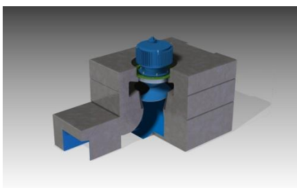
Poldergemaal Elsgeesterpolder
